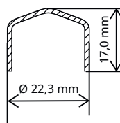
Kolben
