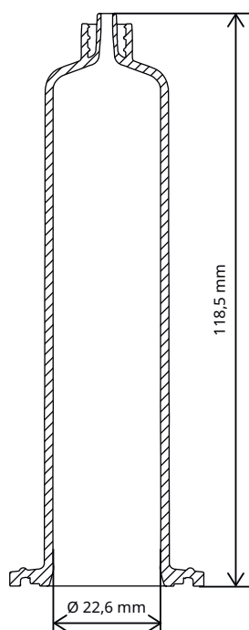
Kartusche
